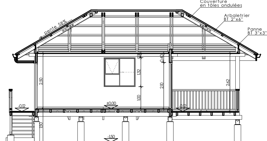
Coupe BB
