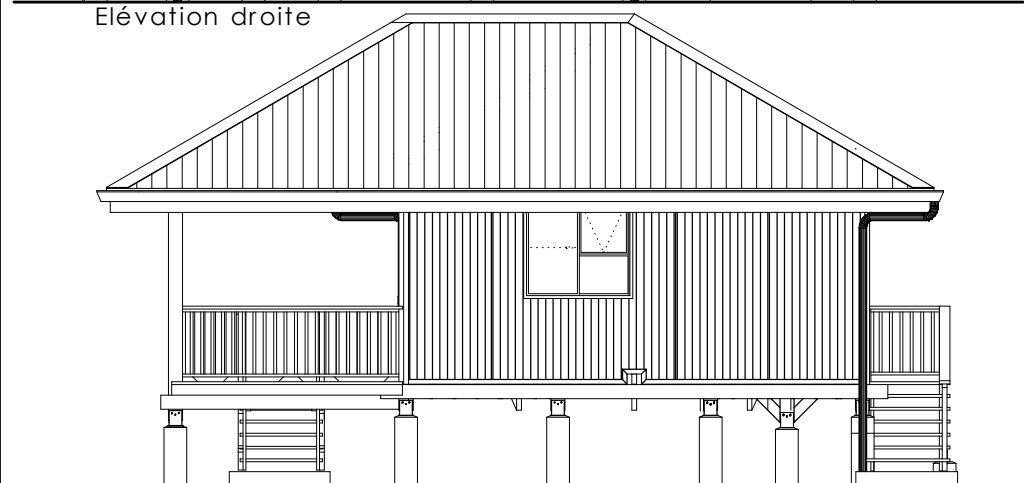
Elévation gauche
