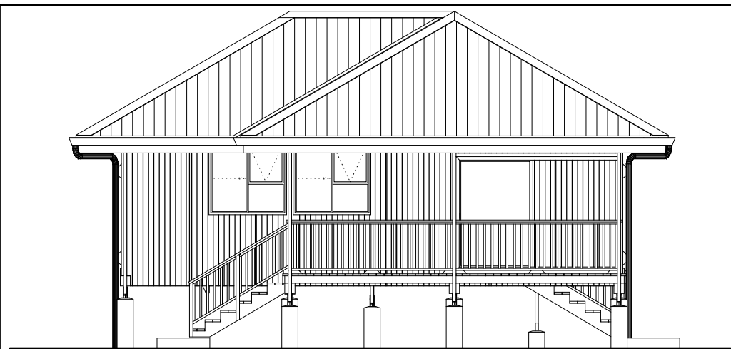
Elévation avant
