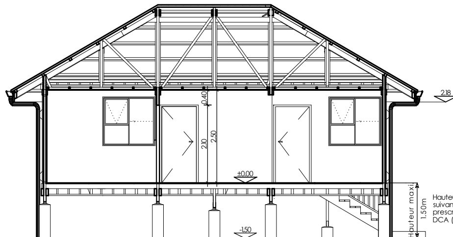
Coupe AA
