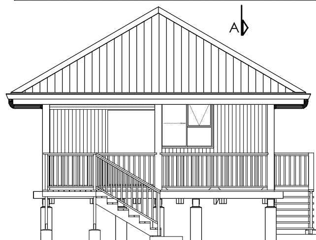
Élévation avant
