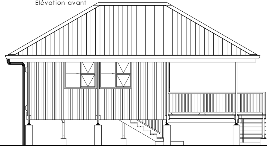
Elévation droite
