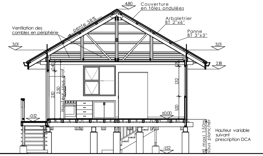
Coupe AA
