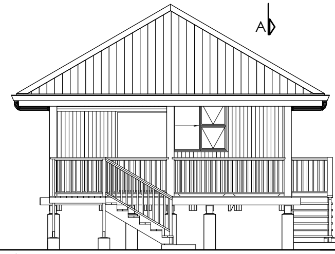
Elévation avant
