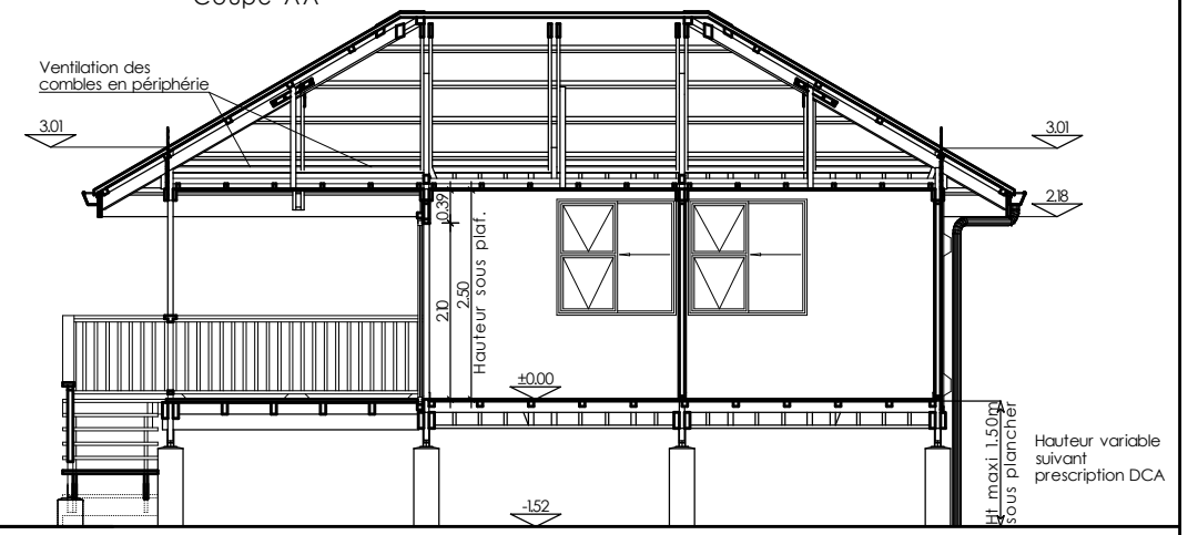
Coupe BB
